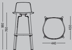
Taburete altura alta Stool high back
