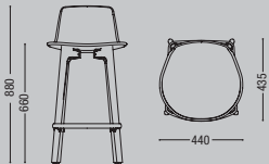
Taburete altura media Stool medium back
